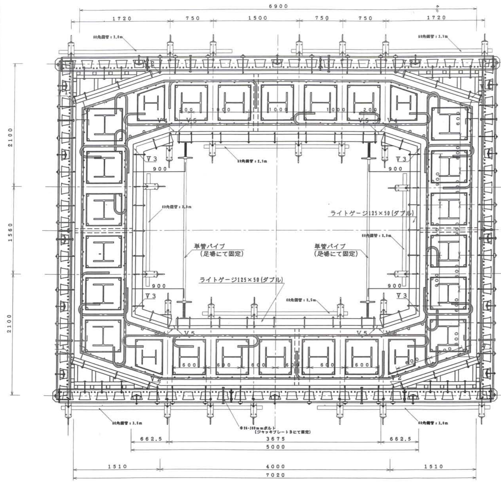
型枠計画図
